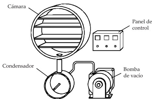
Figura 1. Un dibujo esquemático de los cuatro componentes principales de un liofilizador común.
