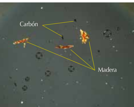
Foto 4: Dispersión con luz transmitida polarizada 10X.
