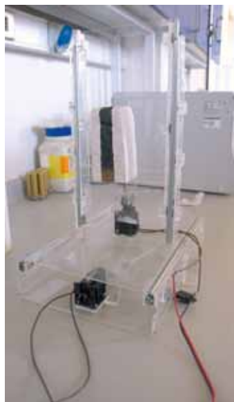
Foto 10: Bloque montado en dispositivo para pruebas de impacto mecánico.
